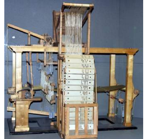
Abb. 11: Der Jacquard-Webstuhl
